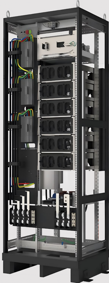
180 kW / 950 DC / 250 A TYP – DR180 / DC Charger Rack (Innenraum)
